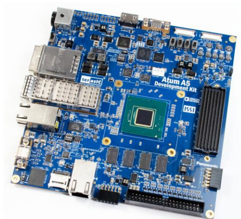
Figure 1-1 Atum A5 board
